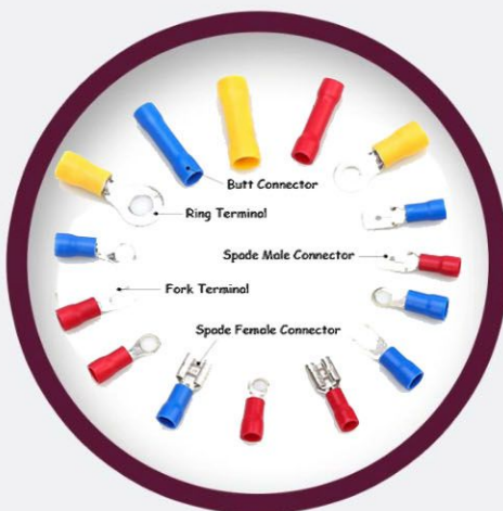
TERMINAL LUGS
